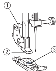
① Адаптер прижимной лапки ② Паз ③ Стержень
