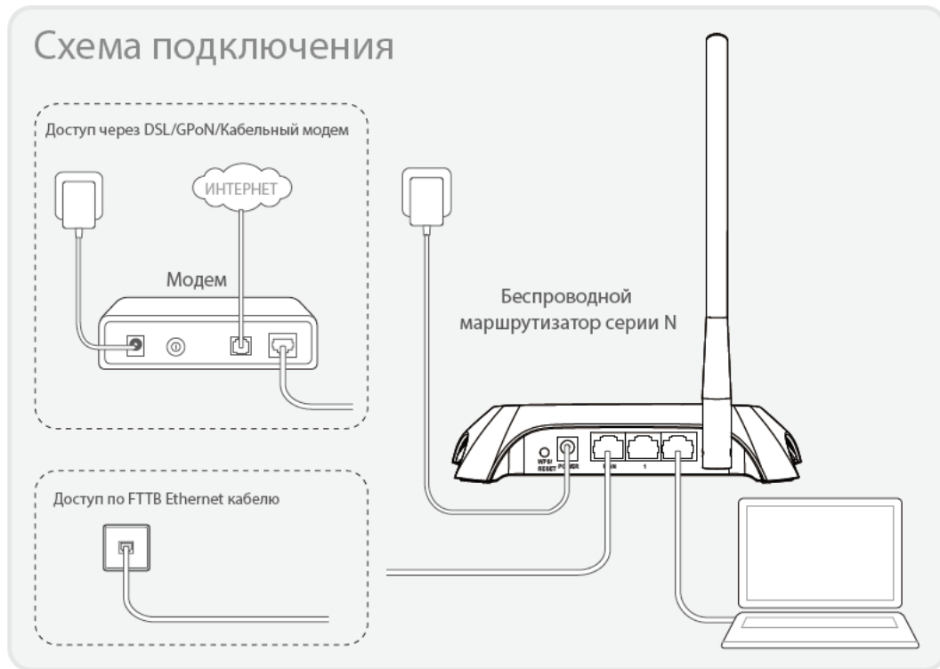
Рис. 2-1 Установка аппаратной части маршрутизатора
