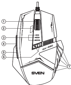
Мал. 1. Вигляд зверху
