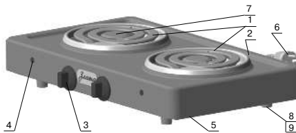
Рисунок 1 — Модель 114Т
