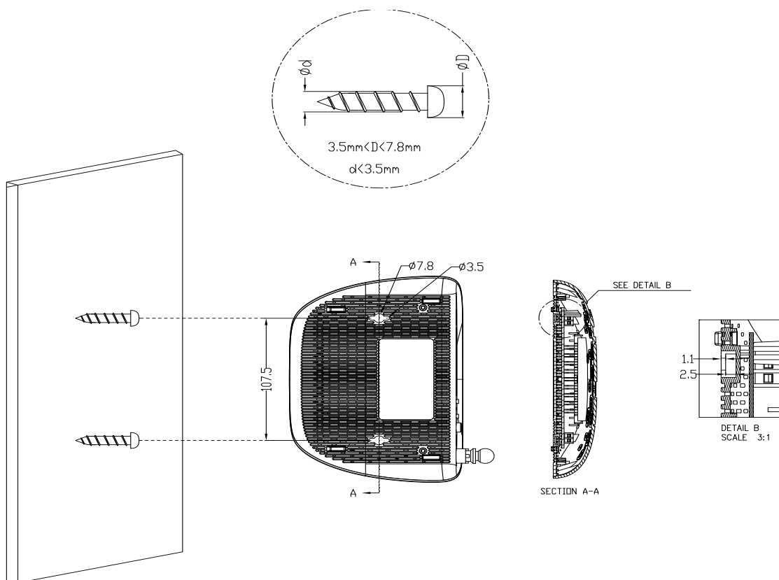
Рисунок 2-1: Настенная установка
