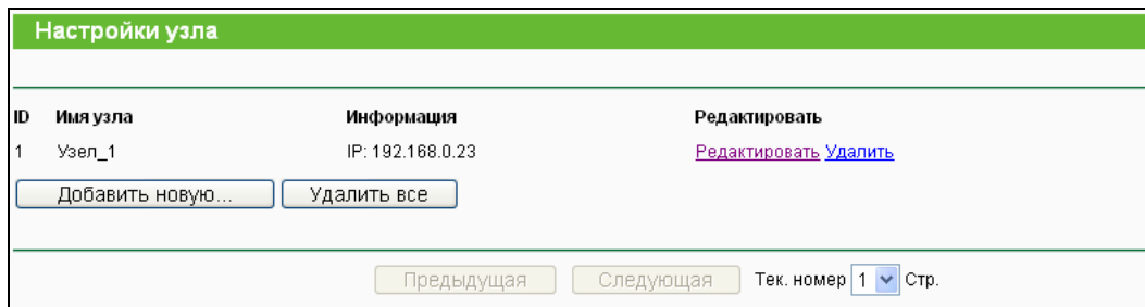
Рис. 4-53 Настройки узла
