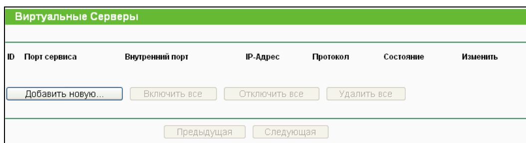
Рис. 4-32 Виртуальные серверы
