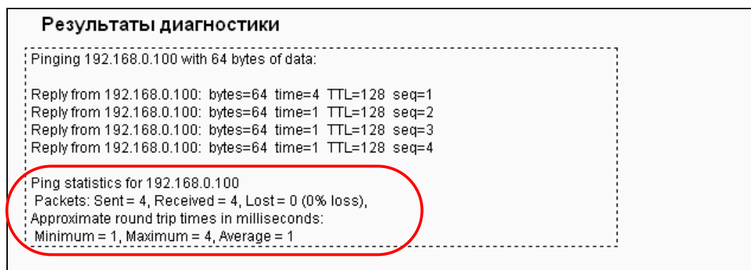
Рис. 4-81 Результаты диагностики
