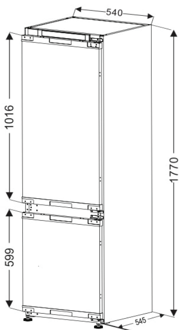
ГАБАРИТЫ МЕБЕЛЬНОГО ФРОНТА И ХОЛОДИЛЬНИКА
