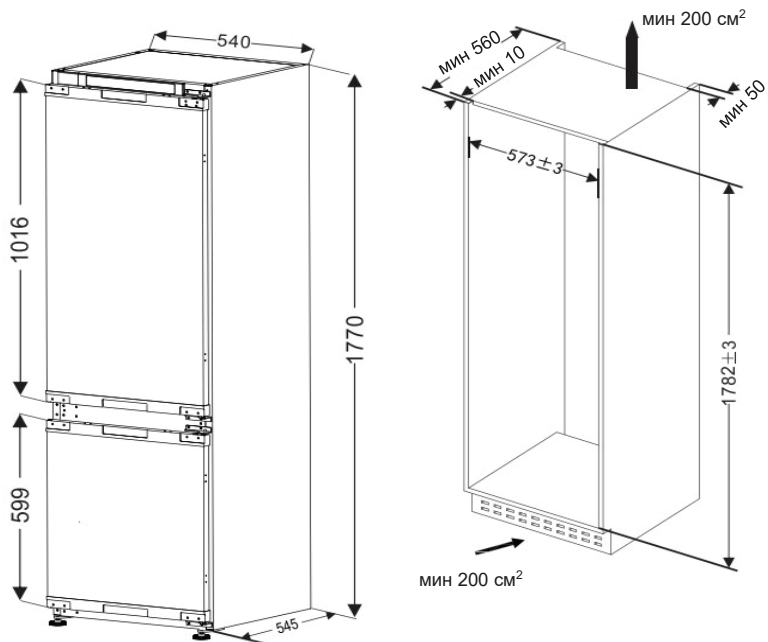
ЖИҢАЗ ФРОНТЫ МЕН ТОҢАЗЫТҚЫШТЫҢ ӨЛШЕМДЕРІ
