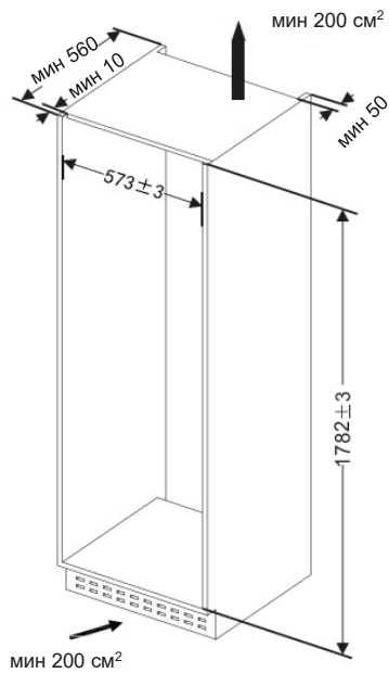
ГАБАРИТЫ МЕБЕЛЬНОГО ФРОНТА И ХОЛОДИЛЬНИКА
