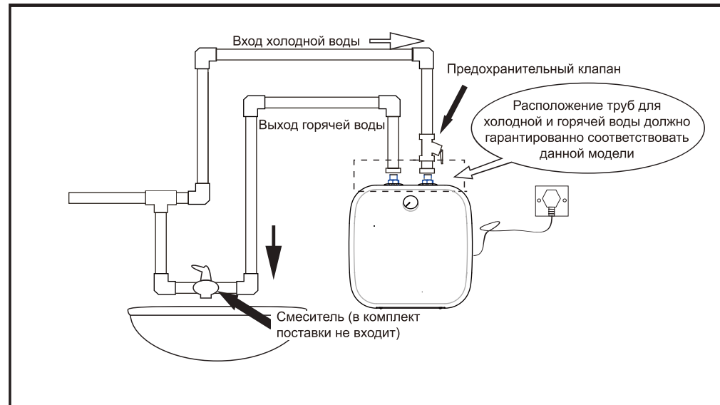
Монтажная схема для моделей, как серии SQ2, у которых горячая вода поступает навехр.
